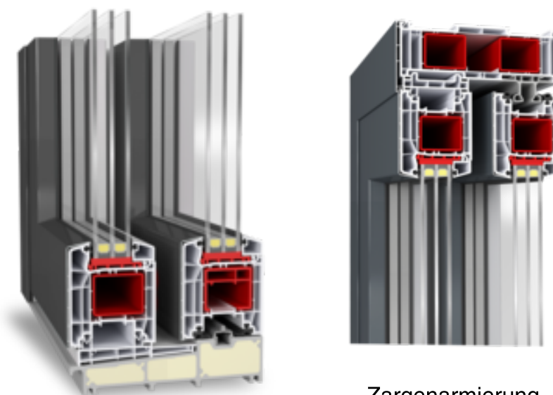
Zargenarmierung
